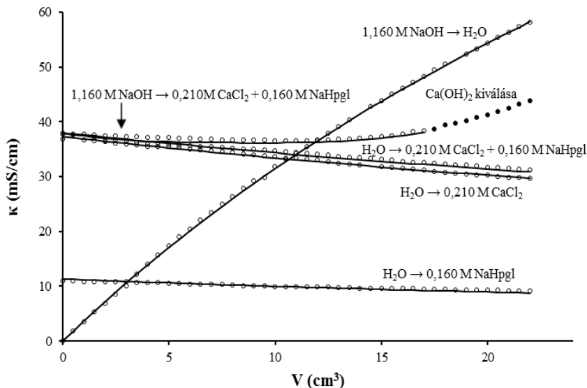
3. ábra: A \text{Ca}^{2+}/\text{Hpgl}^- rendszer konduktometriás titrálási görbéi ( T = (25,0 \pm 0,2)^\circ\text{C} ). A nyilak bal oldalán a titráló, jobb oldalán a titrált oldatok összetétele látható. Az üres körök a mért, míg a folytonos vonalak a számolt értékeket jelölik. A teli körök a csapadékkiválás tartományát jelzik.
